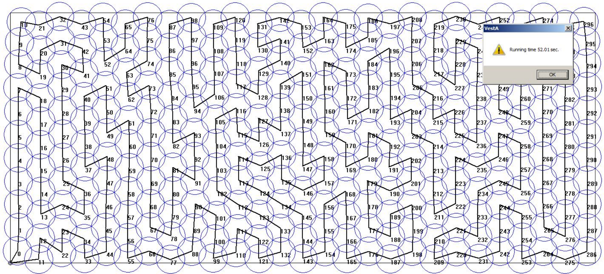
Рисунок В.22 – Покриття 297 колами радіусу 4500 області з розмірами 70000 на 30000 – після оптимізації довжини траси кільцевого типу
