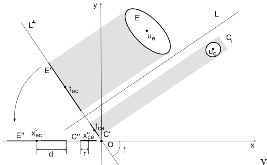
Рисунок 2.7 – Побудова квазі \rho -функції \Phi'^{CE}(v_c, u_e, f)
