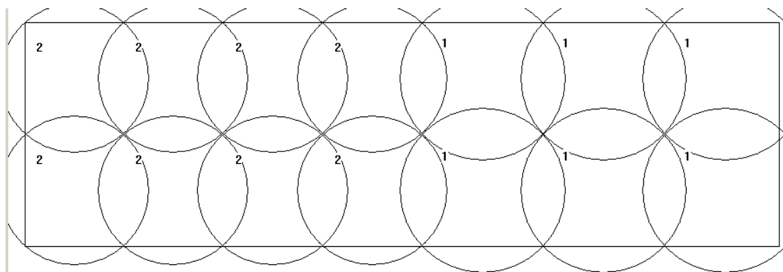
Рисунок В.12 – Результат розв'язання задачі секційно-регулярного покриття області з розмірами 100x30 колами радіуса 11 і 10
