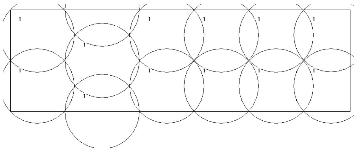
Рис. В.9 – Результат розв'язання задачі секційно-регулярного покриття області з розмірами 100x30 колами радіуса 11
