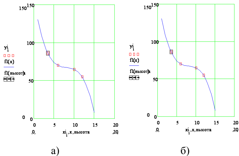
Рисунок 2.3 – Інтерполяція залежності площі, що захищається, від висоти приміщення: а) – для димових ПС при квадратичній схемі; б) – для димових ПС при трикутній схемі
