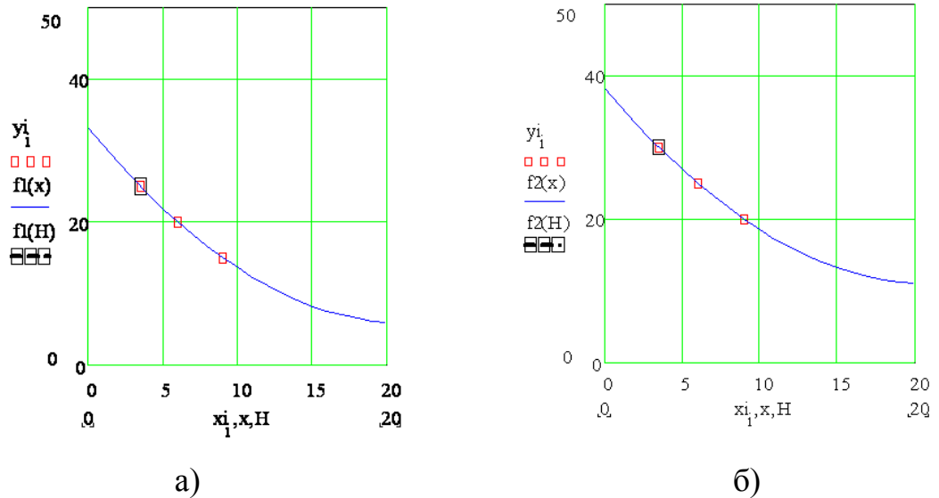
Рисунок 2.2 – Інтерполяція залежності площі, що захищається, від висоти приміщення: а) – для теплових ПС при квадратичній схемі; б) – для теплових ПС при трикутній схемі
