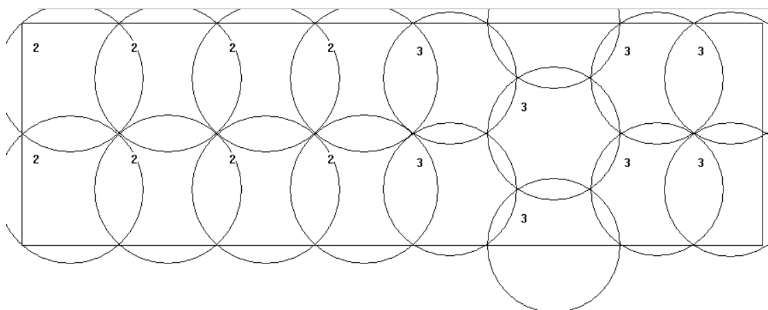
Рисунок В.14 – Результат розв'язання задачі секційно-регулярного покриття області з розмірами 100x30 колами радіуса 9 і 10
