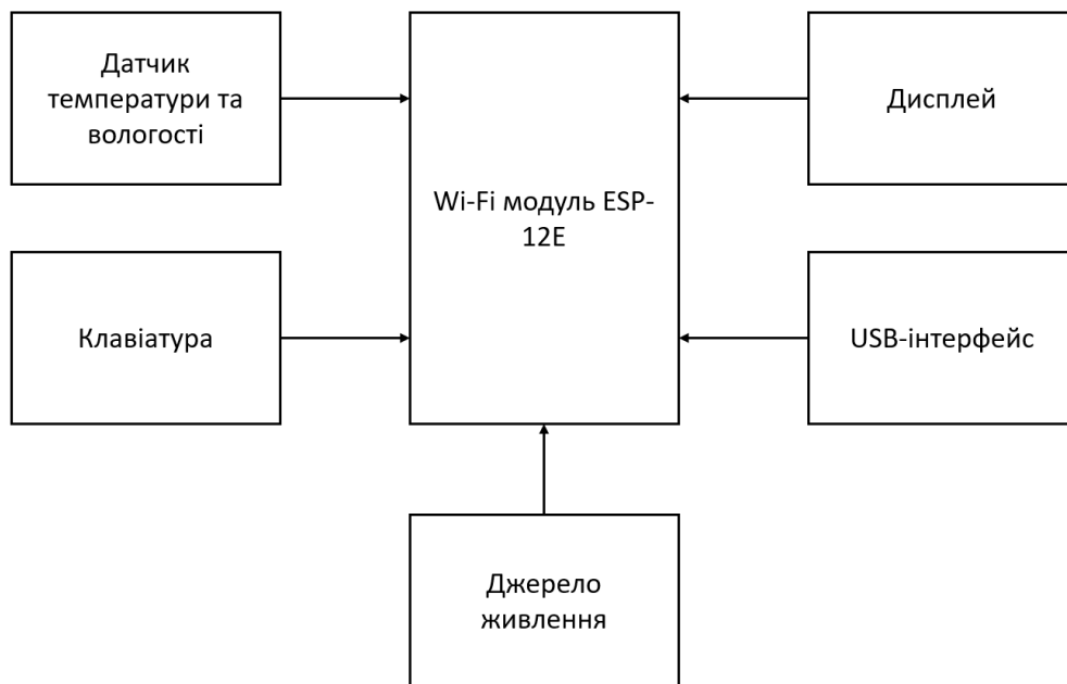
Рисунок 1 – Блок-схема приладу
