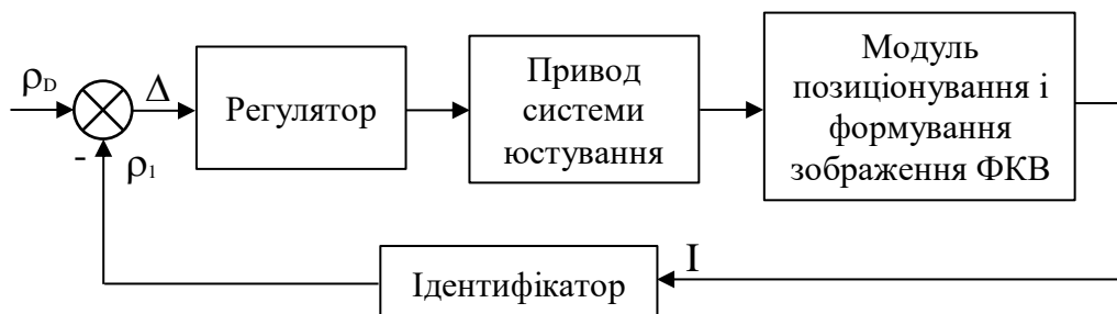
Рисунок 3.11 – Функціональна схема процесу позиціонування за однією координатою
