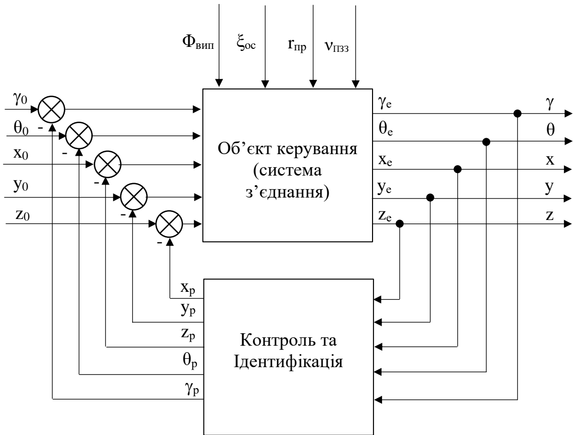
Рисунок 2.2 – Загальна схема керування процесом з'єднання ФКВ
