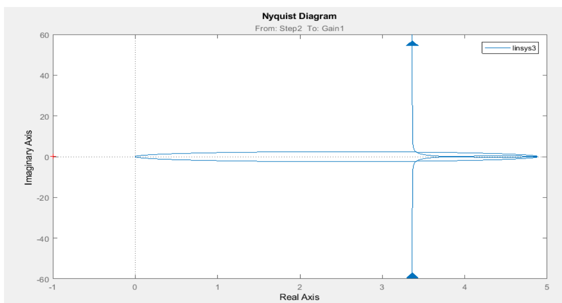
Рисунок 3.16 – Діаграма Найквіста
