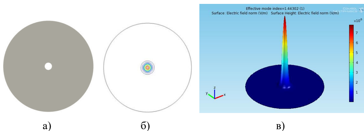
Рисунок 4.6 – Одномодове ОВ з радіусом серцевини r = 5 \text{ мкм} (а) та розподіл поля основної моди на довжині хвилі \lambda = 1,55 \text{ мкм} (б, в)
