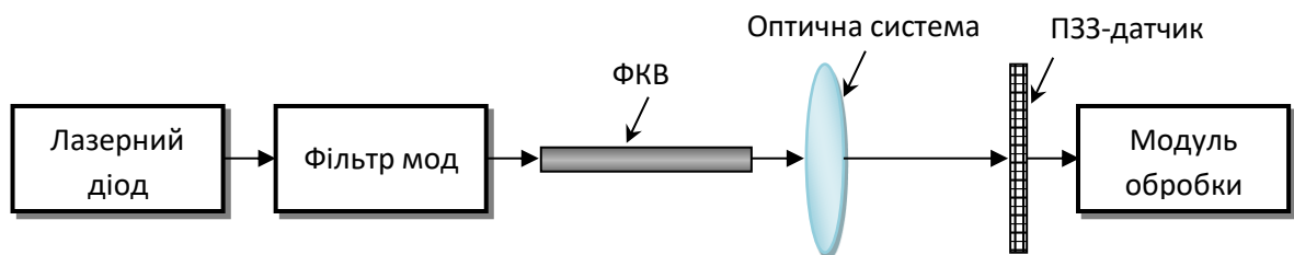
Рисунок 5.20 – Схема вимірювання ФКВ методом ближнього поля
