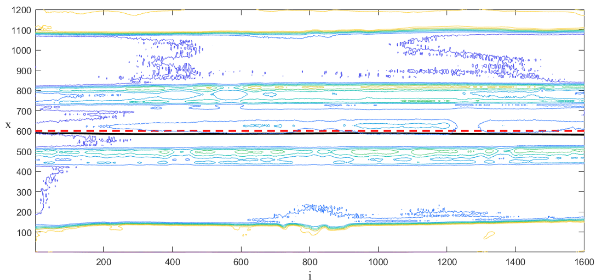
Рисунок 5.18 – Розрахована методом автозгортки (суцільна лінія) та інтегральним методом (переривчаста лінія) вісь ФКВ, зображеного на рис. 5.2, a
