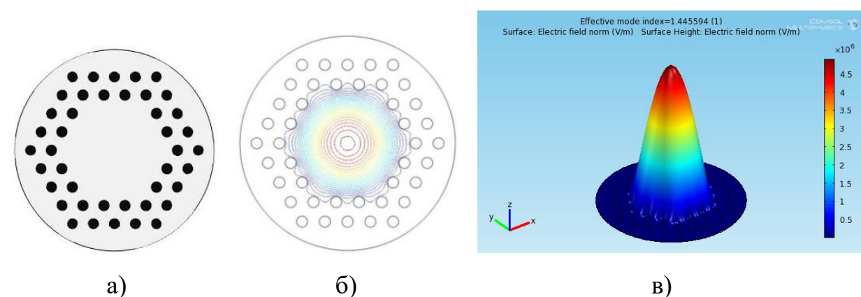
Рисунок 4.5 – ФКВ з діаметром серцевини 60 мкм (а) та отриманий розподіл поля основної моди на довжині хвилі \lambda = 1,55 мкм (б, в)
