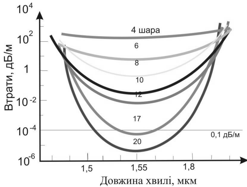
Рисунок 1.17 – Залежність втрат на тунелювання від довжини хвилі для різної кількості періодичних шарів в ФКВ
