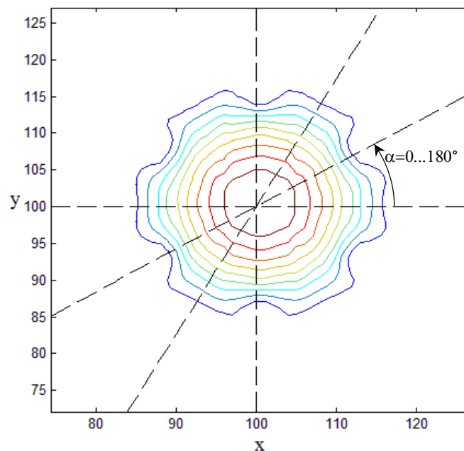
Рисунок 4.24 – Лінії (перетини), що проходять через центр модового поля ФКВ, визначений методом автозгортки
