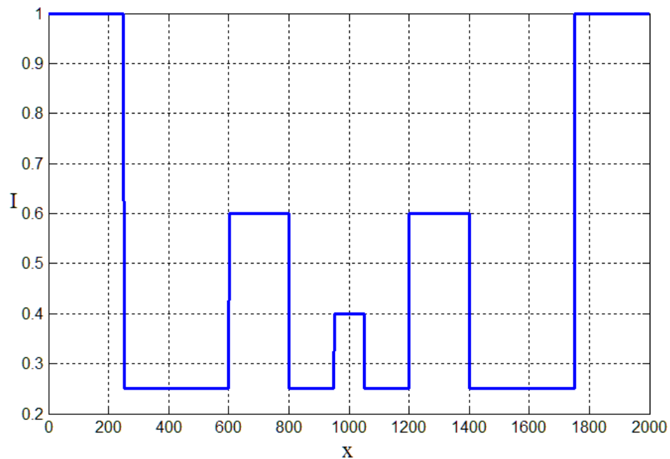
Рисунок 3.5 – Вихідний розподіл інтенсивності оптичного поля
