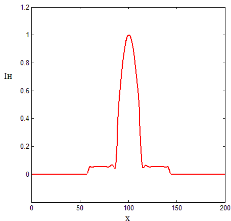
Рисунок 4.27 – Згладжений розподіл інтенсивності модового поля ФКВ після фільтрації
