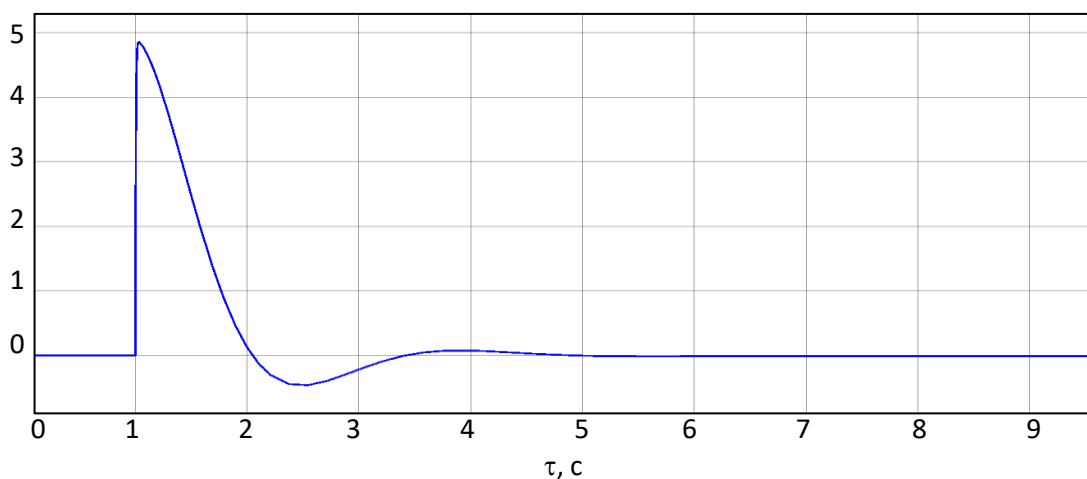
Рисунок 3.13 – Перехідна характеристика системи позиціонування
