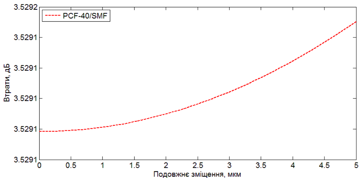
Рисунок 4.12 – Залежність втрат від подовжнього зміщення в з'єднанні фотонно-кристалічного волокна з радіусом серцевини 19,7 мкм та одномодового оптичного волокна
