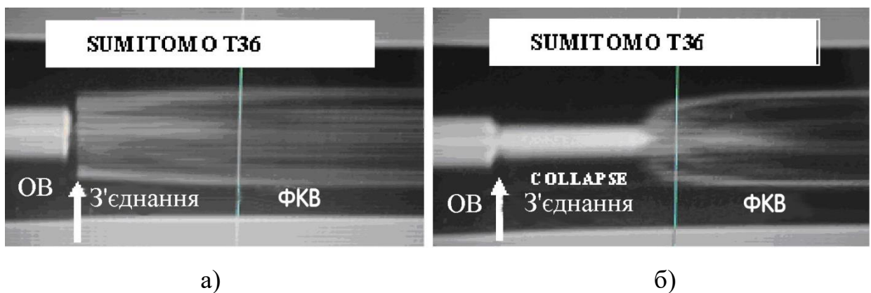
Рисунок 1.10 – З'єднання ФКВ та одномодового волокна:
