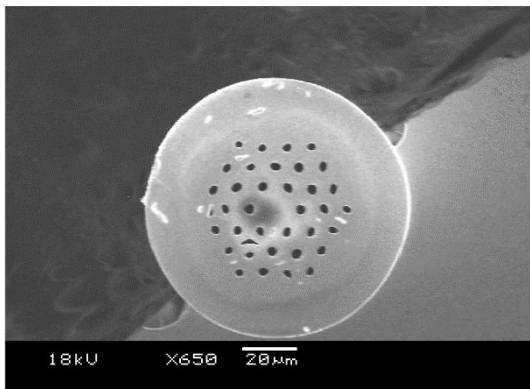
Рисунок 1.14 – Зображення поперечного перетину ФКВ з d/D = 0,388 та D = 8,5 \text{ мкм} (а); зображення місця з'єднання ФКВ і ОВ (б)
