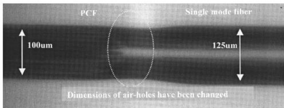
Рисунок 1.13 – З'єднання ФКВ та стандартного ОВ
