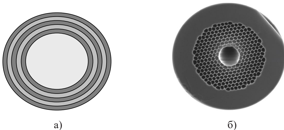
Рисунок 1.3 – Поперечні перетини ФКВ:
