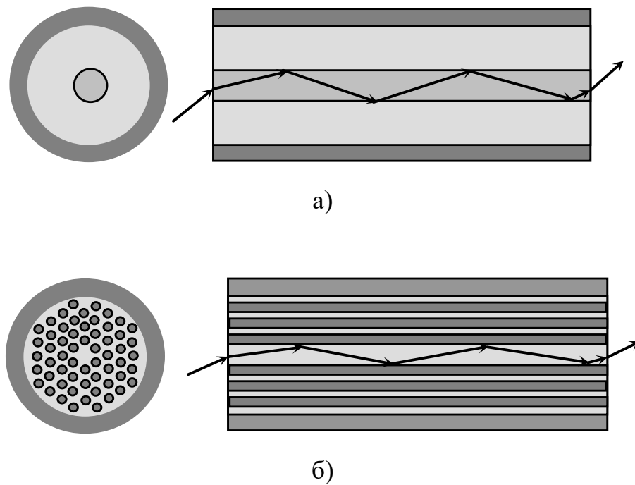
Рисунок 1.2 – Поперечні перетини та хід світлових промінів в стандартному оптоволокні (а) та фотонно-кристалічному волокні (б)
