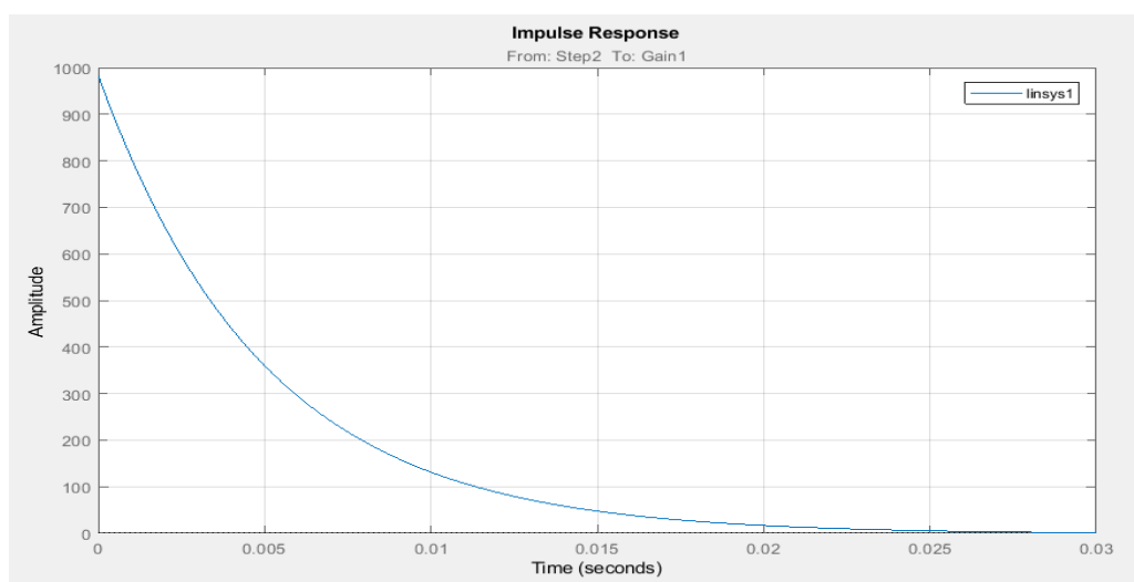
Рисунок 3.14 – Імпульсна характеристика системи позиціонування
