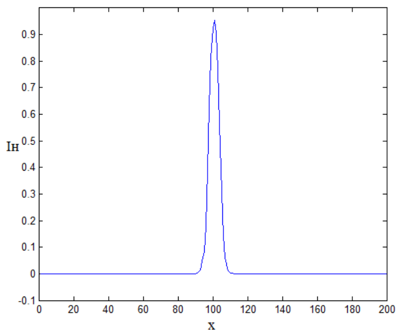
Рисунок 4.26 – Одномірний розподіл інтенсивності випромінювання одномодового оптичного волокна
