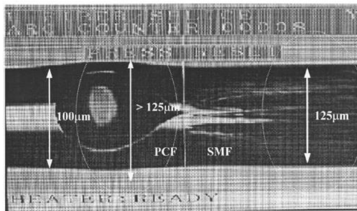
Рисунок 1.11 – Ріст пухиря у процесі зварювання електричною дугою
