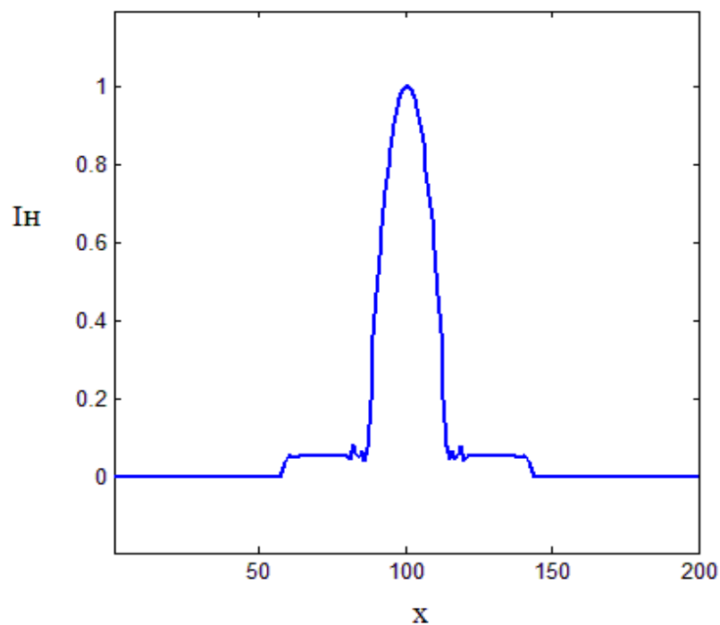
Рисунок 4.25 – Розподіл інтенсивності випромінювання ФКВ в перетині \alpha=0^\circ
