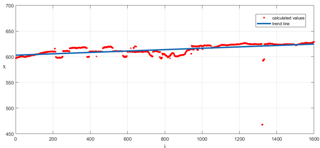
Рисунок 5.14 – Розрахований центр серцевини ФКВ, зображеного на рис. 5.2, а (переривчаста лінія) та лінія тренду (суцільна лінія)
