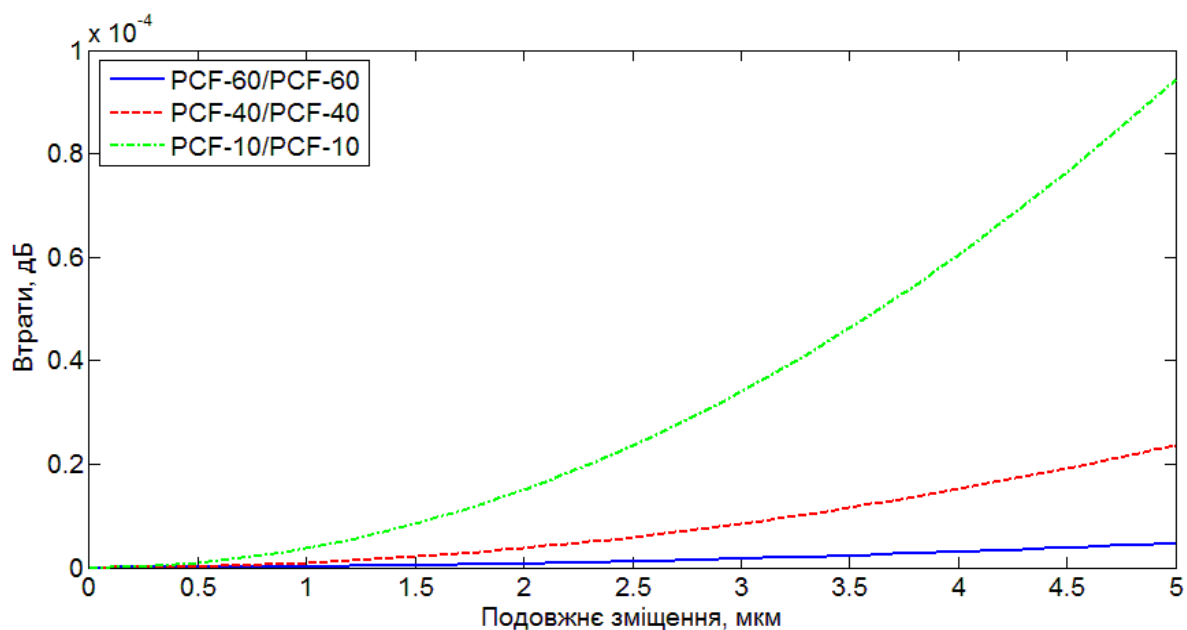
Рисунок 4.14 – Залежність втрат від поздовжнього зміщення в з'єднаннях ідентичних фотонно-кристалічних волокон
