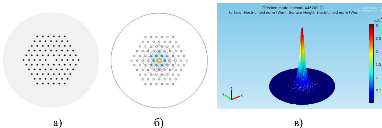
Рисунок 4.3 – Структура ФКВ з діаметром серцевини 10 мкм (а) та отриманий розподіл поля основної моди на довжині хвилі \lambda = 1,55 мкм (б, в)
