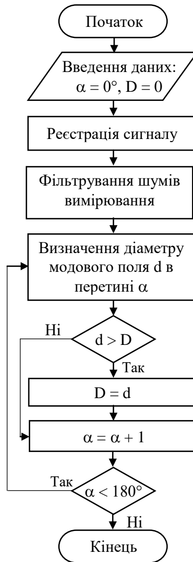
Рисунок 4.20 – Алгоритм визначення максимального діаметру модового поля в поперечному перетині ФКВ
