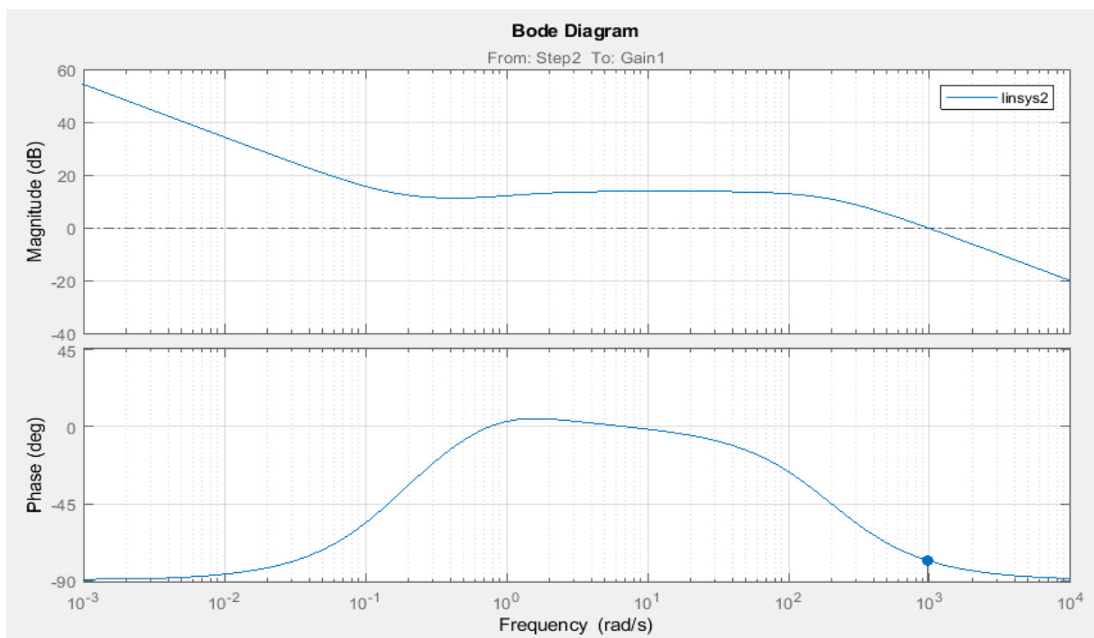
Рисунок 3.15 – АЧХ і ФЧХ системи позиціонування
