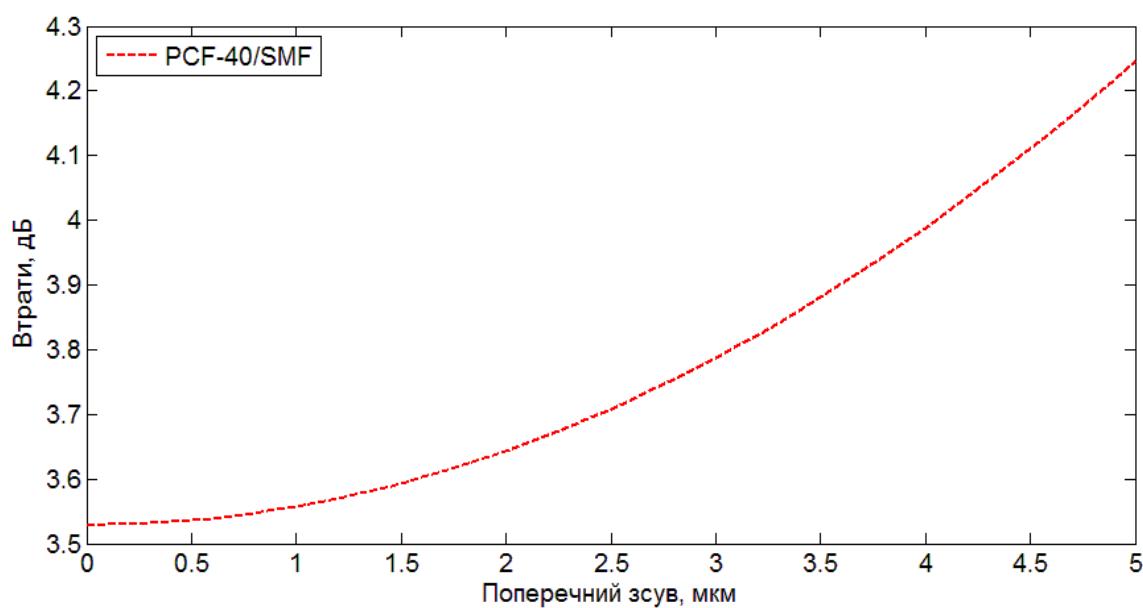
Рисунок 4.7 – Залежність втрат від поперечного зсуву в з'єднанні фотонно-кристалічного волокна з радіусом серцевини 5 мкм та одномодового оптичного волокна
