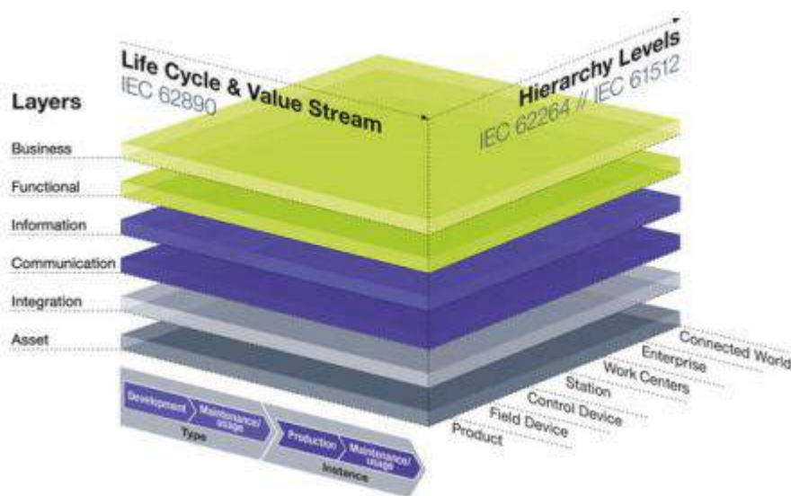
Рисунок 1.5 –Архітектурна модель Industry 4.0 (RAMI 4.0) [143,144]
