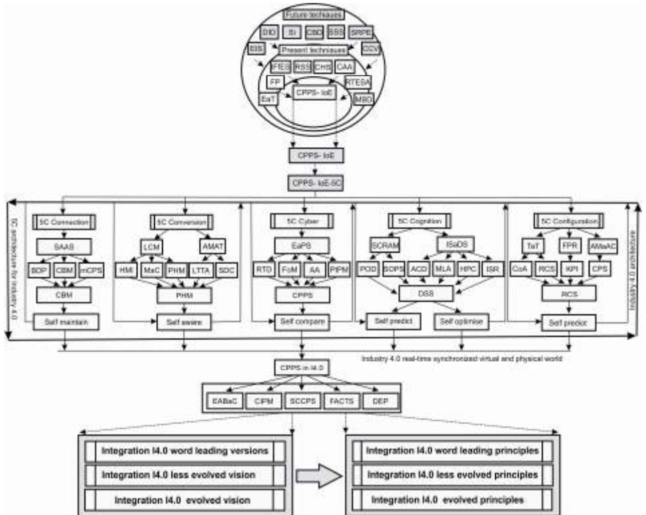
Рисунок 1.11 – Фрагмент імперичної архітектурної моделі інтеграції CPPS-IoE в архітектурі 5C для Industry 4.0 [164]
