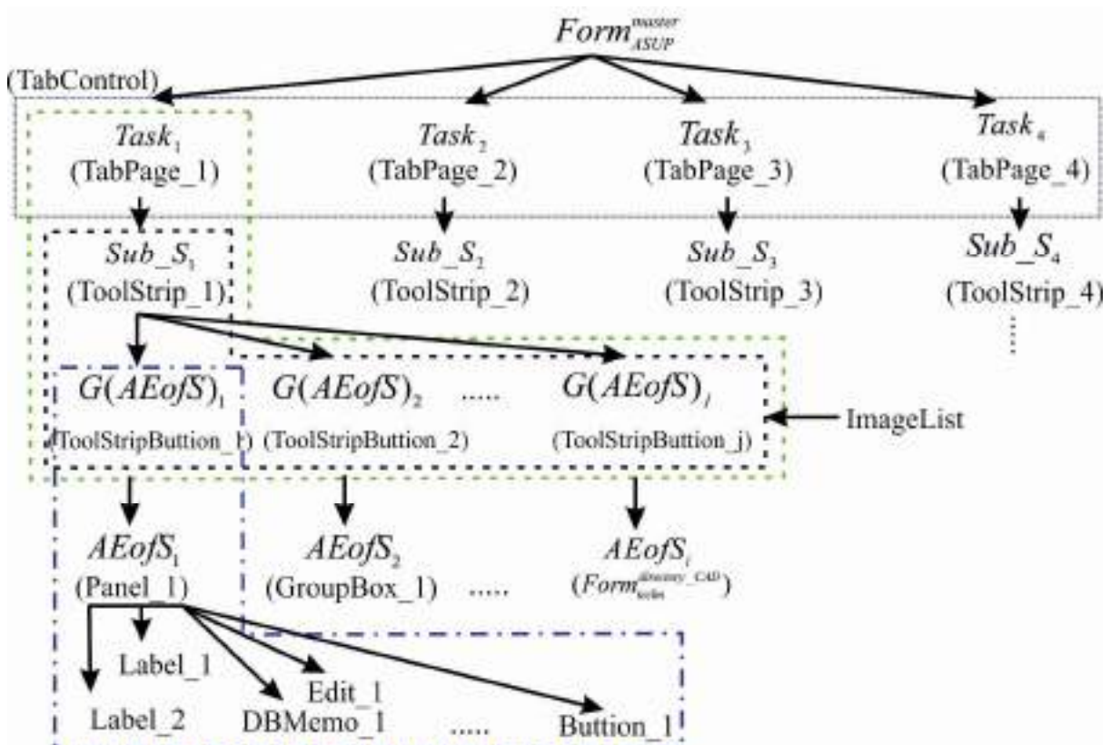
Рисунок 6.22 – Граф реалізації GUI «Основного меню управління»
