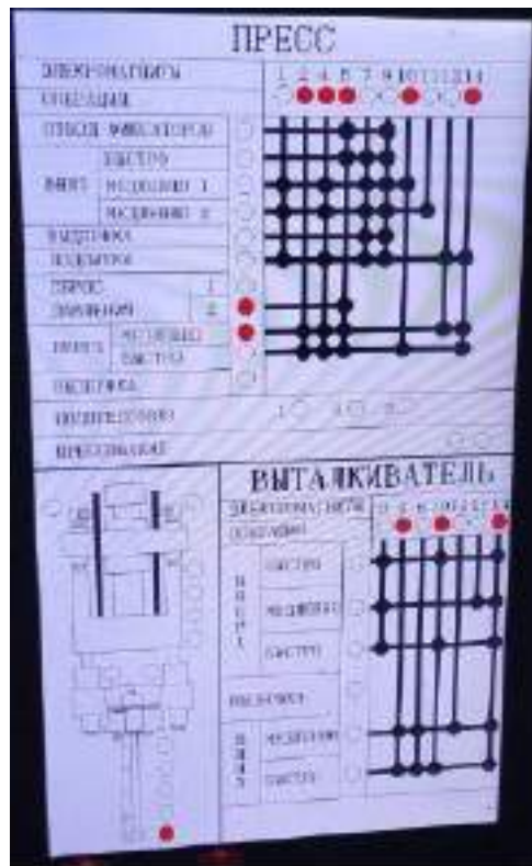
Рисунок 6.36 – Мнемосхема преса ДА2238Б
