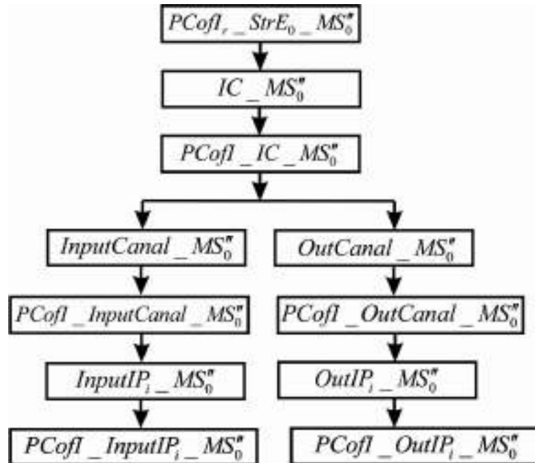
Рисунок 2.11 – Дерево рішень декомпозиції на інфологічному етапі
