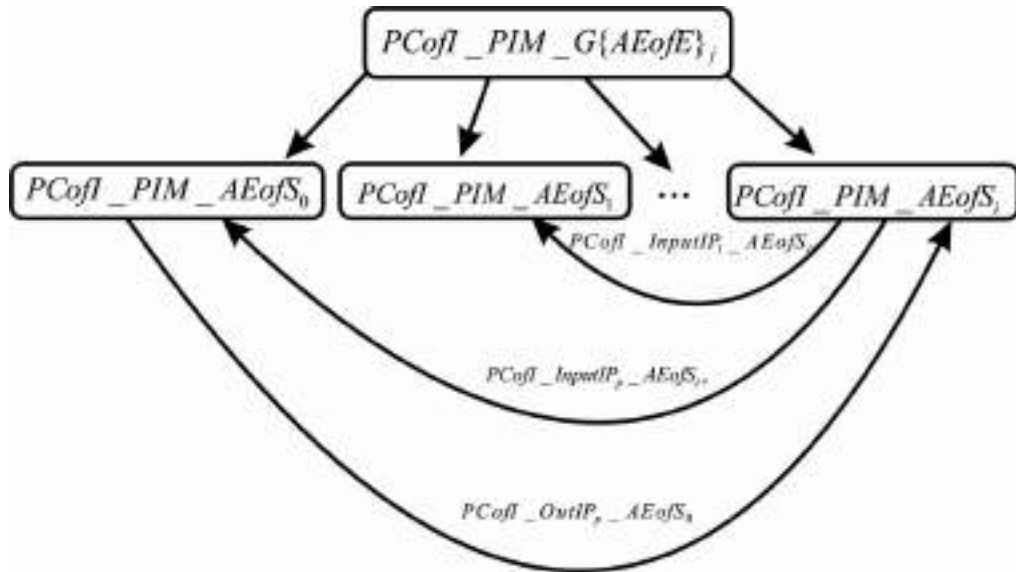
Рисунок 3.6 – Графова системна модель інформаційного етапу на рівні декомпозиції PCofl\_PIM\_G\{AEofE\}_i
