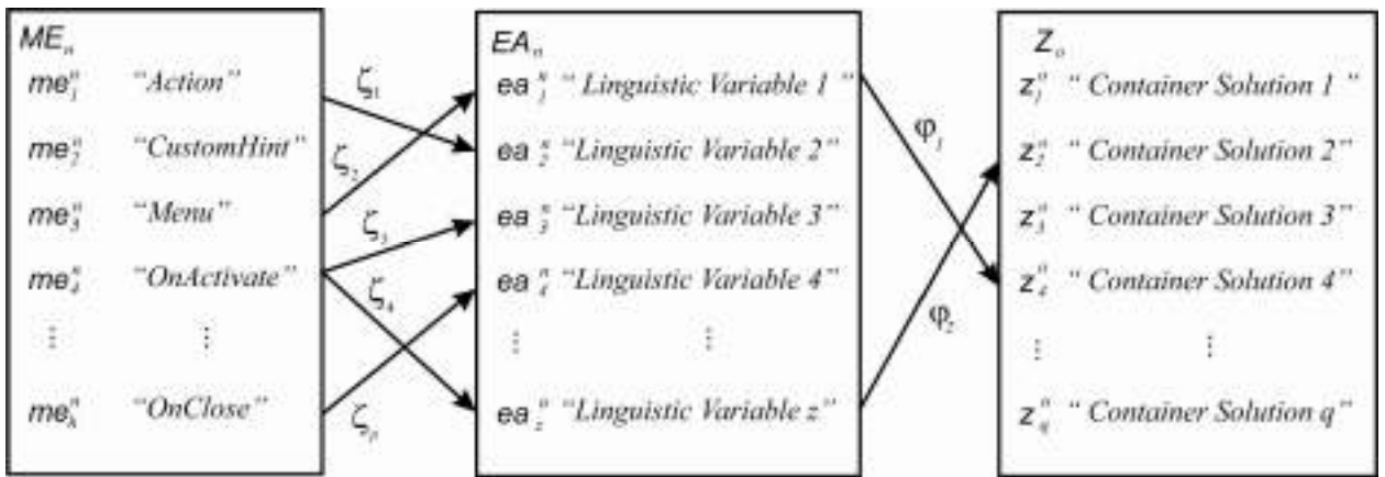
Рисунок 4.6 – Приклад взаємодії множин (me_1^n, \dots, me_h^n) \in ME_n за допомогою «Lingustic Variable» (ea_1^n, \dots, ea_z^n) \in EA_n і множини (z_1^o, z_2^o, \dots, z_q^o) \in Z_o «Container Solution»
