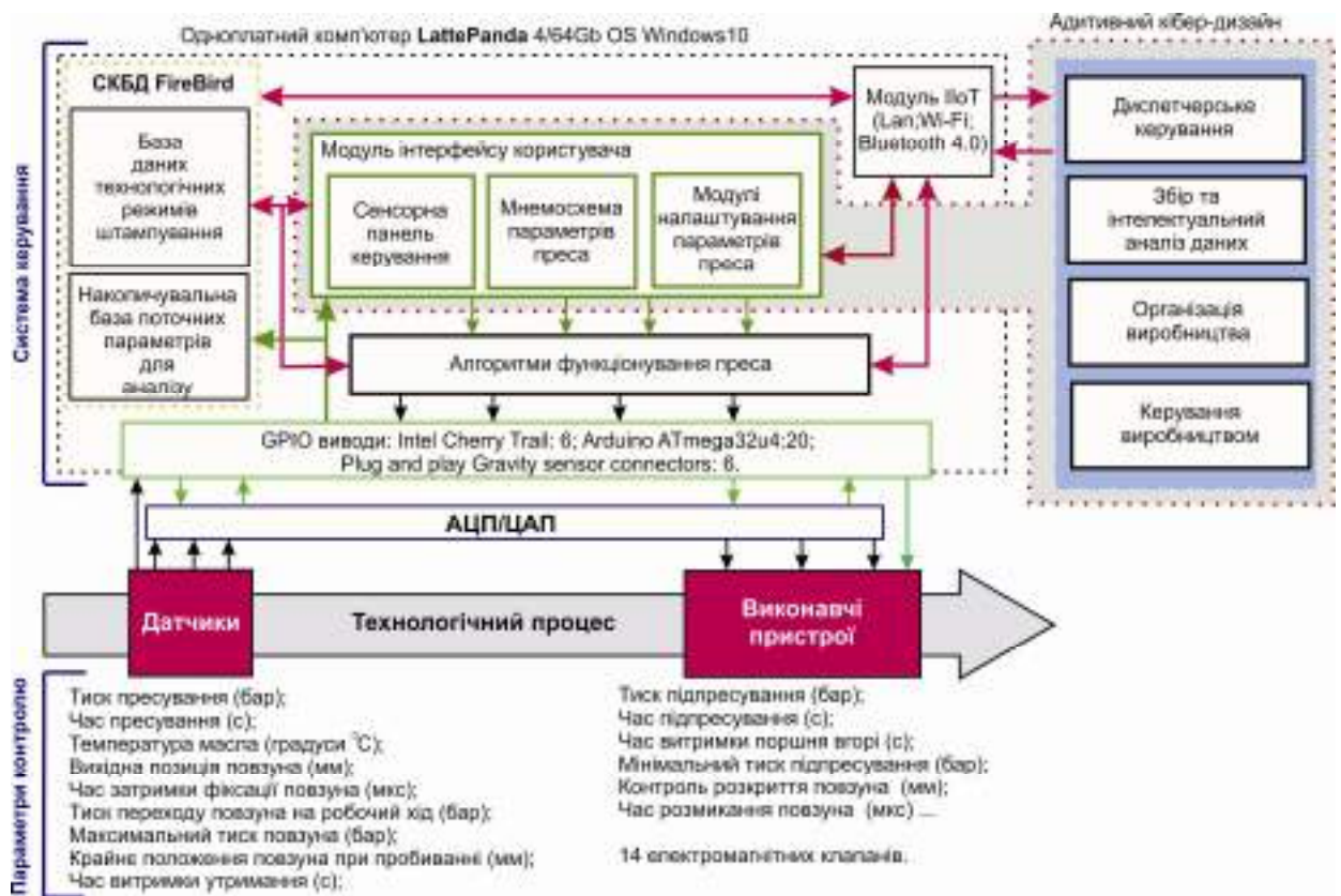
Рисунок 6.38 – Структура модернізованого преса DA2238B на базі LattePanda 4/64Gb
