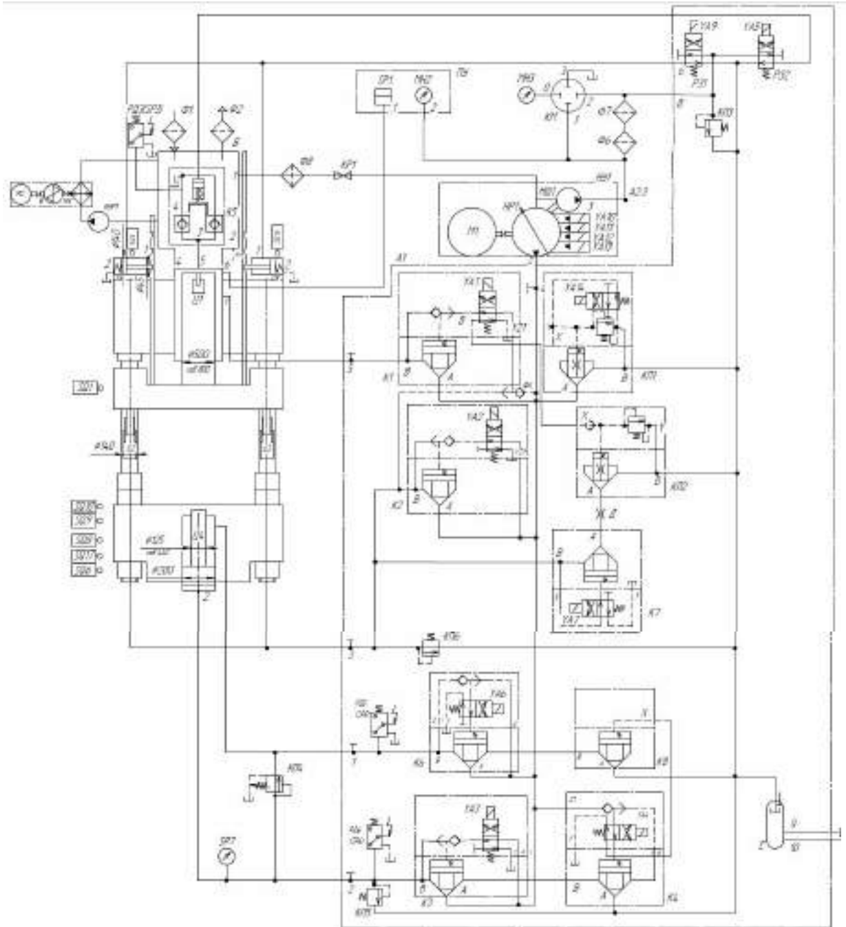
Рисунок 6.33 – Схема гідравлічна принципова преса ДА2238Б
