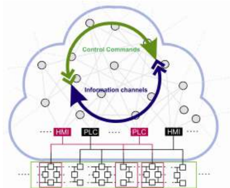
Рисунок 1.20 – Представлення кібернетичної складової CPPS
