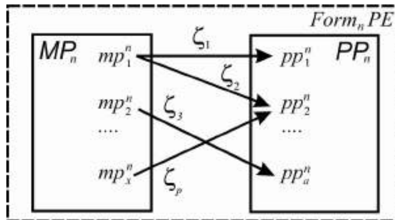
Рисунок 4.5 – Відповідність другого окремого випадку (коли параметру mp_x^n може належати множина значень pp_a^n )
