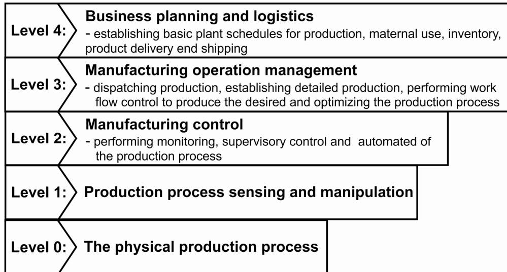
Рисунок 1.7 – Архітектура ISA-95 (S95) [157]
