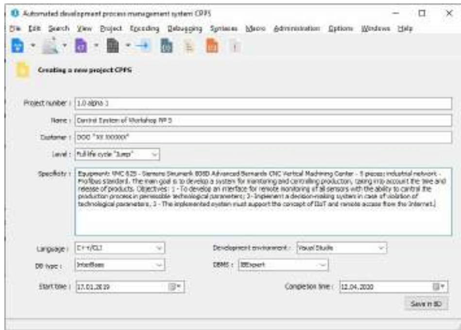
Рисунок 6.13 – Вікно модуля «New project CPPS»
