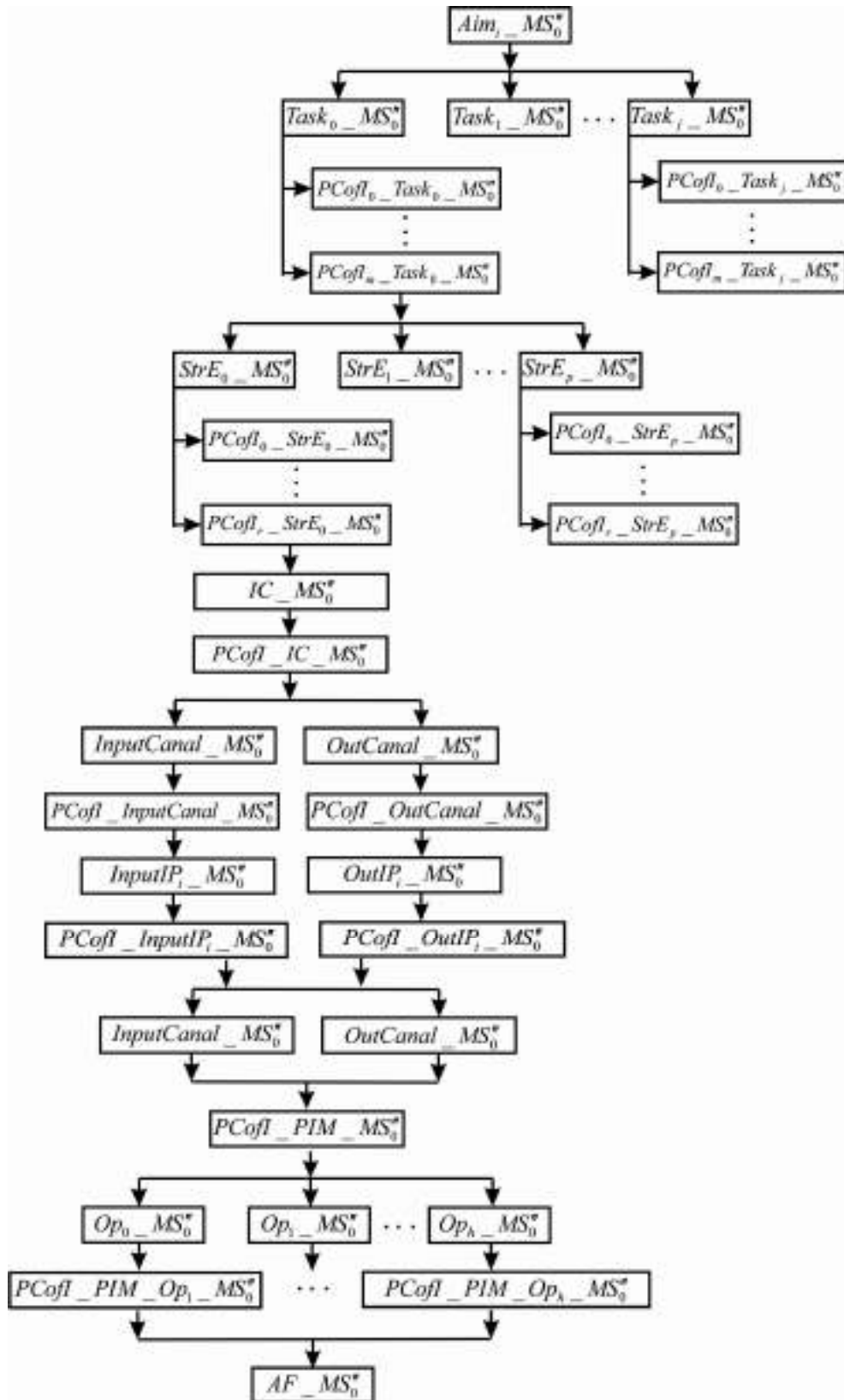
Рисунок 2.14 – Дерево рішень декомпозиції рівня MS_0''
