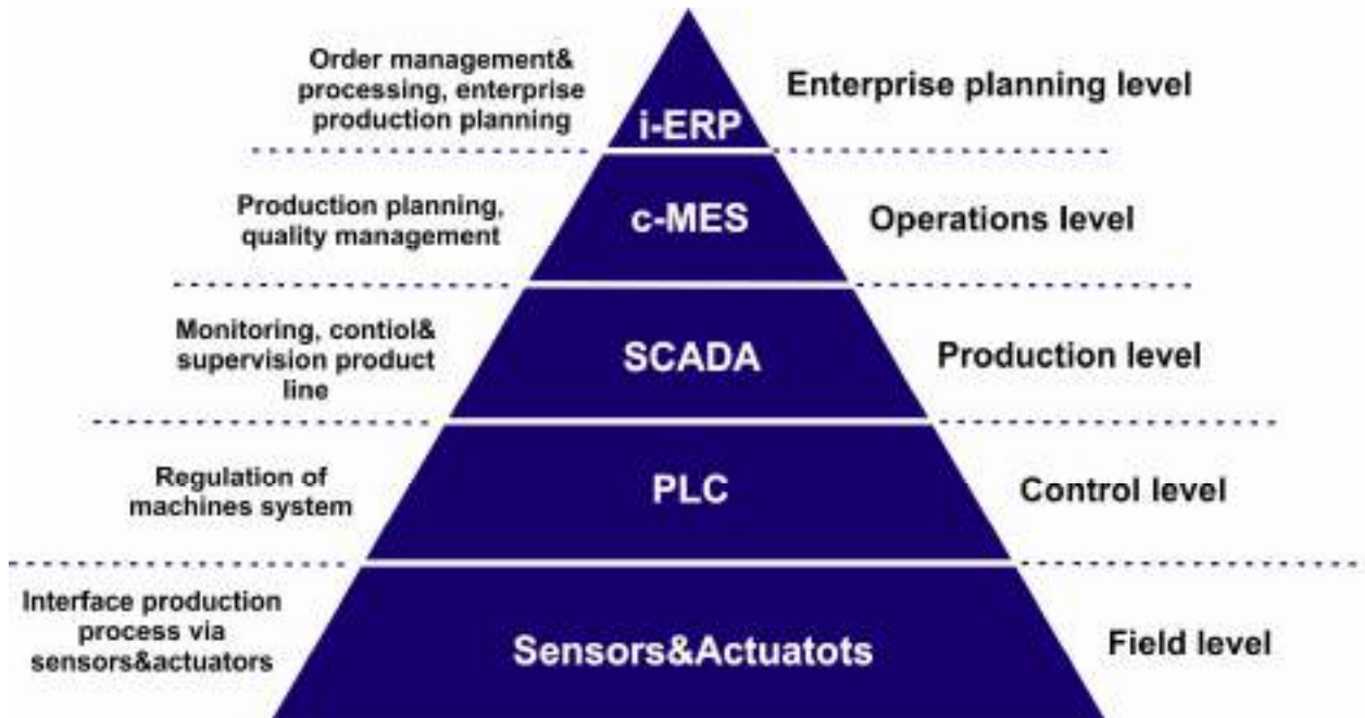
Рисунок 1.10 – Інтерпретація моделі DIKW для вертикальної інтеграції ієрархічних рівнів CPPS
