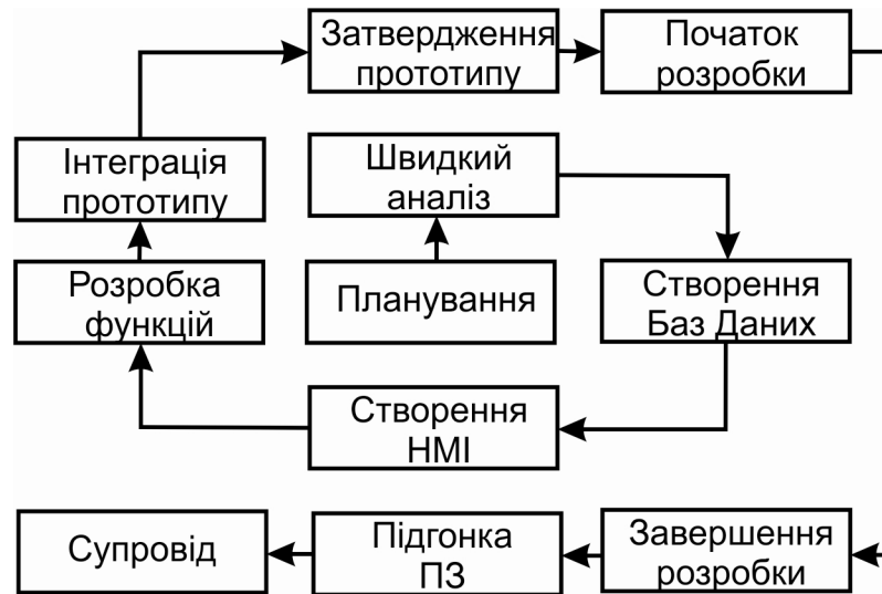
Рисунок 1.16 – Модель прототипування
