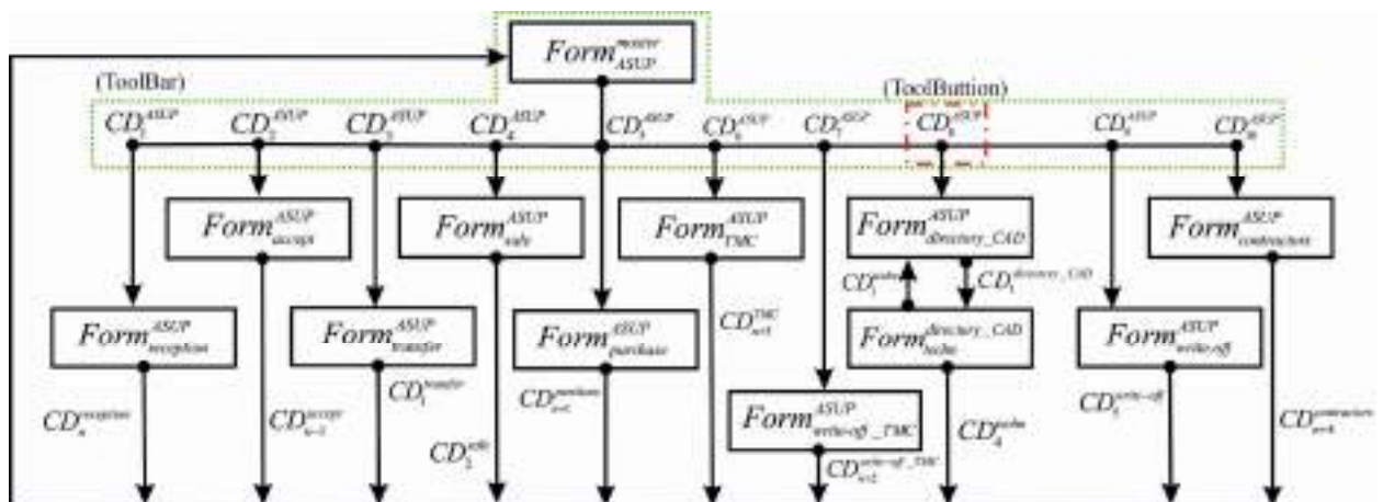
Рисунок 6.21 – Графічна модель структури зв'язків Windows Forms в «OSCEM»
