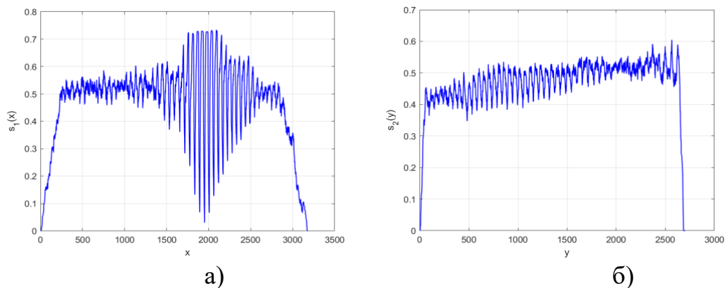
Рисунок 6 – Графіки усереднення для проєктивно спотвореного зображення b :
