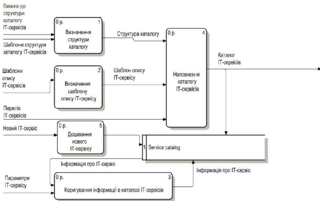
Рис.2. Діаграма потоків даних задачі формування каталогу ІТ-сервісів
