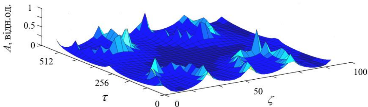
Рисунок 3.27 – Залежність амплітуди імпульса від кількості проходів по резонатору \zeta і тривалості \tau , при \alpha_1 = 45^\circ, \alpha_2 = 88^\circ, \theta = 90^\circ (рис.3.6) або при подачі на РК-комірку, замість півхвильової пластини, напруги 9,8 В.
