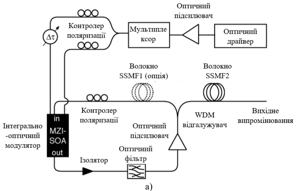
Рисунок 1.11 – Зображення кільцевого волоконного лазера з активною синхронізацією мод: а) схема лазера;
