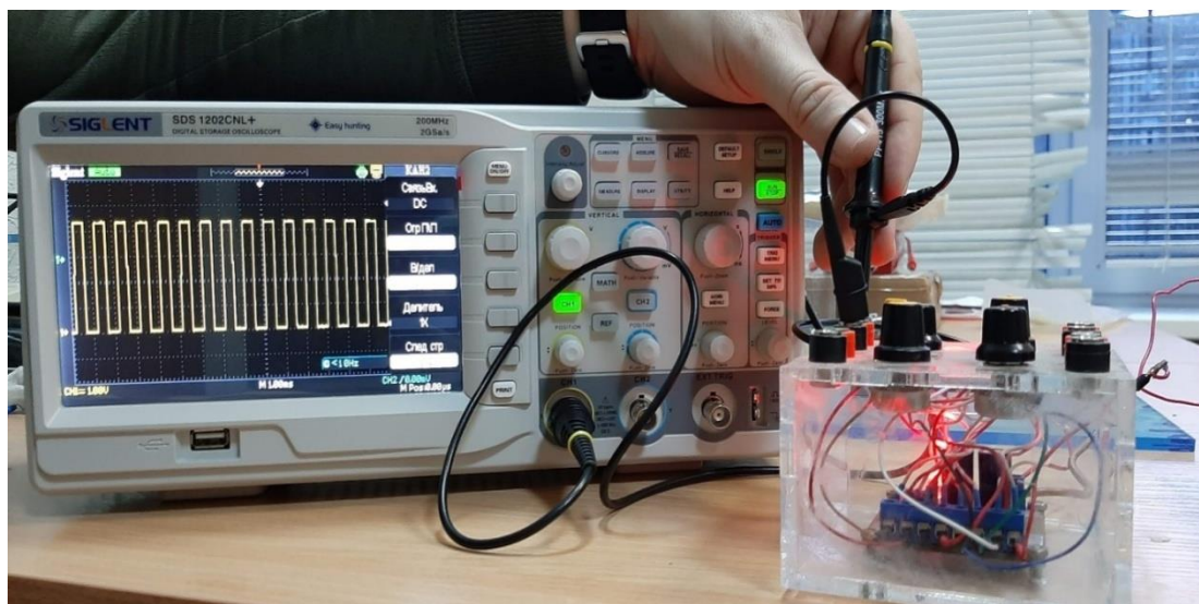
Рисунок 4.11 – Фото дослідження системи управління РК-комірками
