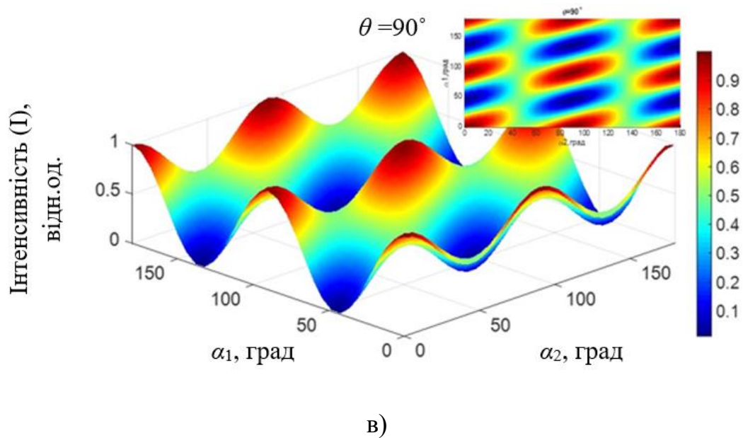
Рисунок 3.6, аркуш 2: в) \theta = 90^\circ
