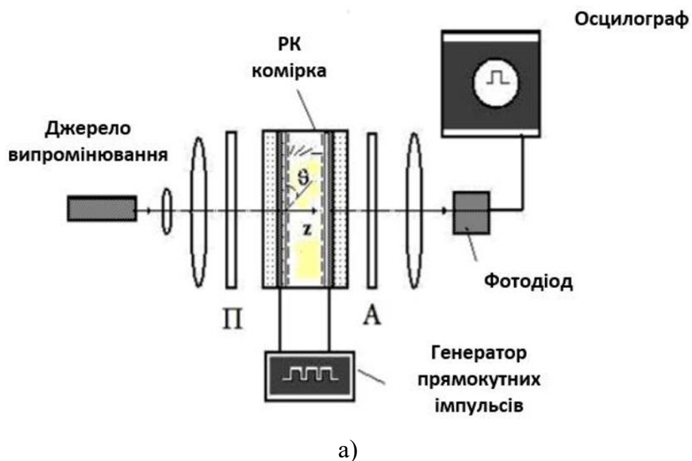
Рисунок 3.12 – Вимірювання характеристик НРК комірок: а) електрооптична схема
