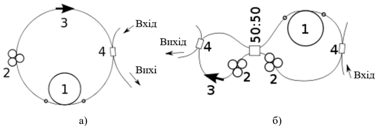
Рисунок 1.9 – Схема кільцевих волоконних резонаторів: а) звичайний кільцевий резонатор, вбудований в волоконний лазер; б) волоконний лазер з синхронізацією мод з кільцевим резонатором у вигляді вісімки; 1 – активне волокно; 2 – поляризатор; 3 – оптичний ізолятор; 4 – WDM-відгалужувач; 50:50 – дільник потужності випромінювання 50/50
