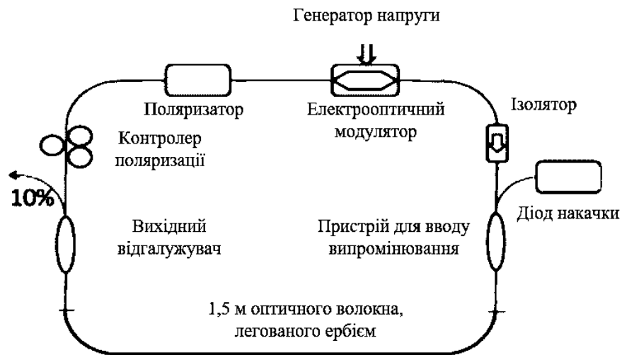
Рисунок 1.15 – Кільцевий волоконний лазер з активною синхронізацією мод
