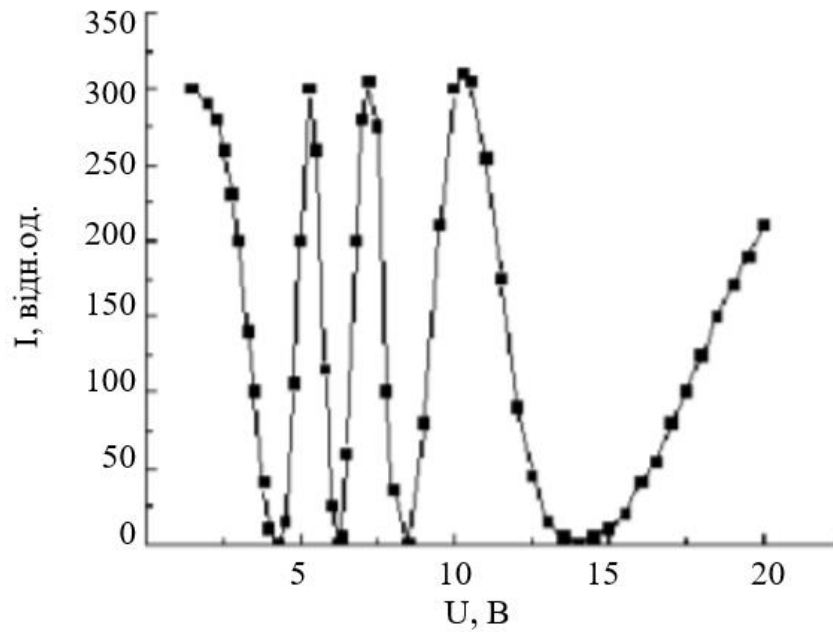
Рисунок 3.13 – Оптичне пропускання РК-комірки в залежності від прикладеної змінної напруги, що подається з частотою 1 кГц [105–106]
