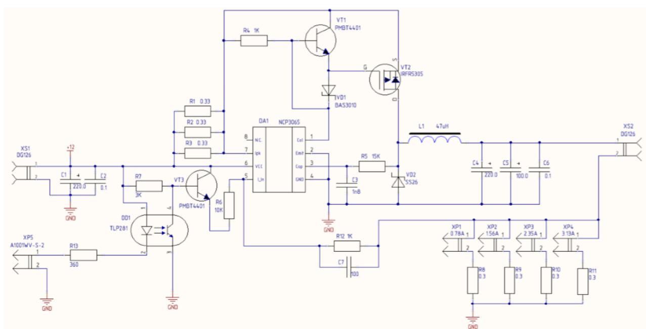
Рисунок 4.5 – Принципова електрична схема системи живлення лазерного діода накачування
