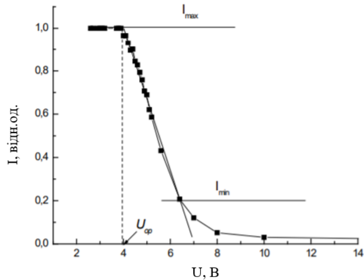
Рисунок 3.20 – Приклад визначення напруг роботи twist комірки [116–119]
