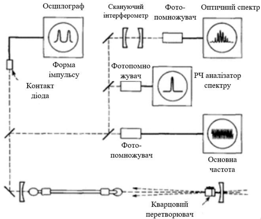
Рисунок 1.10 – Схема реалізації активної синхронізації мод (1964 рік)
