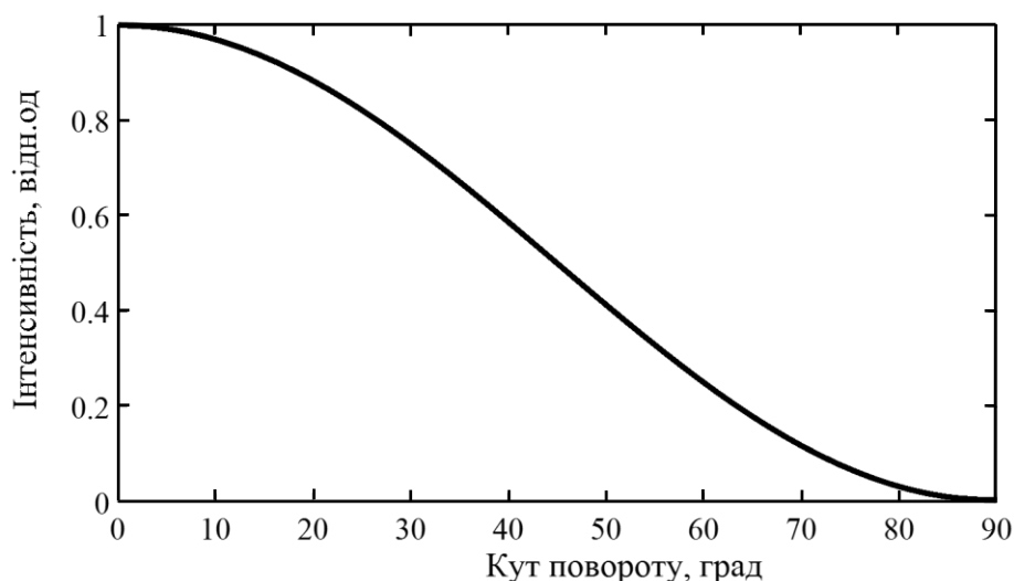
Рисунок 3.19 – Залежність інтенсивності випромінювання, що пройшло через twist -структуру від кута закрутки
