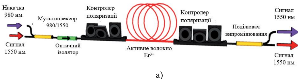
Рисунок 2.3 – Волоконний лазер з нелінійним обертанням поляризації мод:
