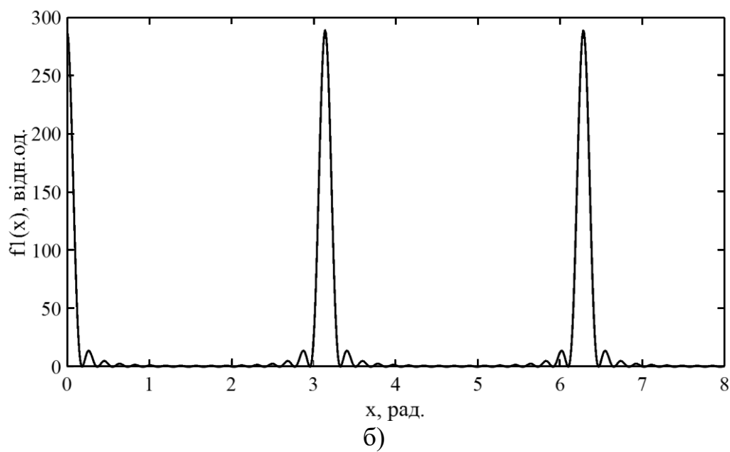
Рисунок 1.4 – Функції: а) (\sin 5x / \sin x)^2 ; б) (\sin 17x / \sin x)^2
