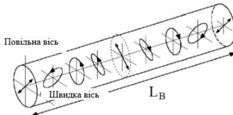
Рисунок 2.1 – Зміна стану поляризації випромінювання в оптичному волокні
