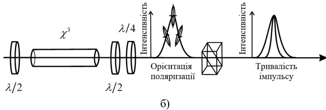
Рисунок 2.3, аркуш 2: б) схема принципу роботи нелінійного обертання поляризації
