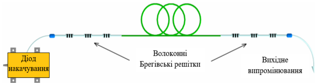
Рисунок 1.8 –Волоконний лазер з бреггівськими дзеркалами
