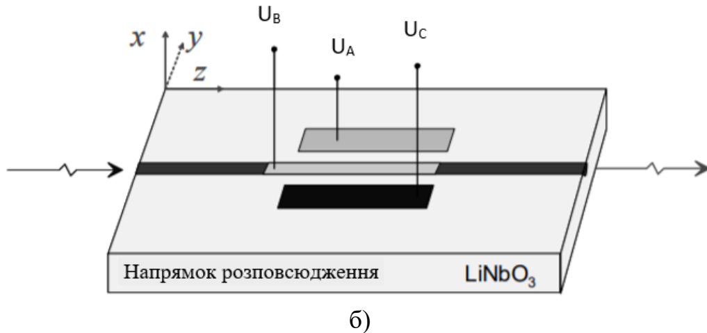
Рисунок 1.11, аркуш 2: б) інтегрально-оптичний модулятор
