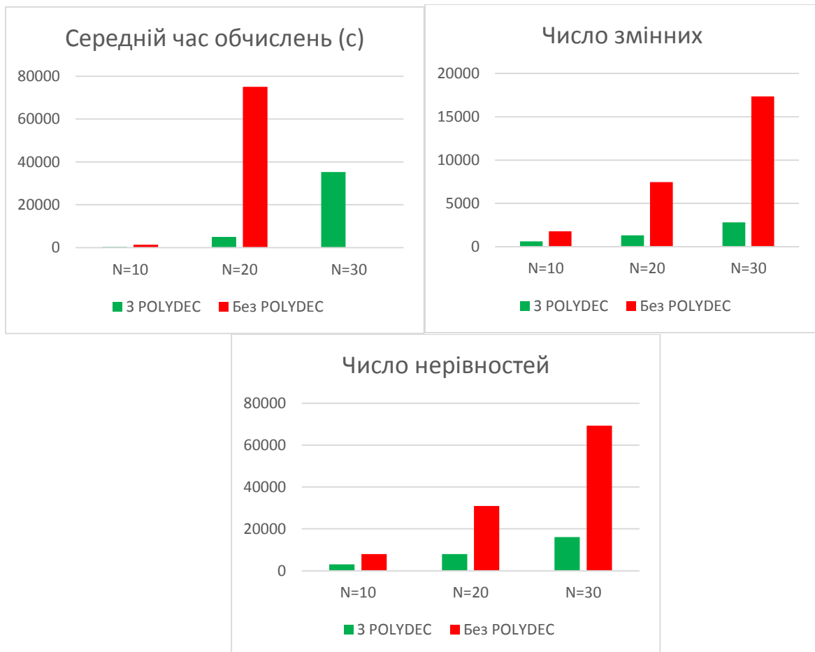
Рисунок 4 – Результати порівняння розв'язання різних задач упаковки довільних багатогранників з застосуванням та без застосування методу
