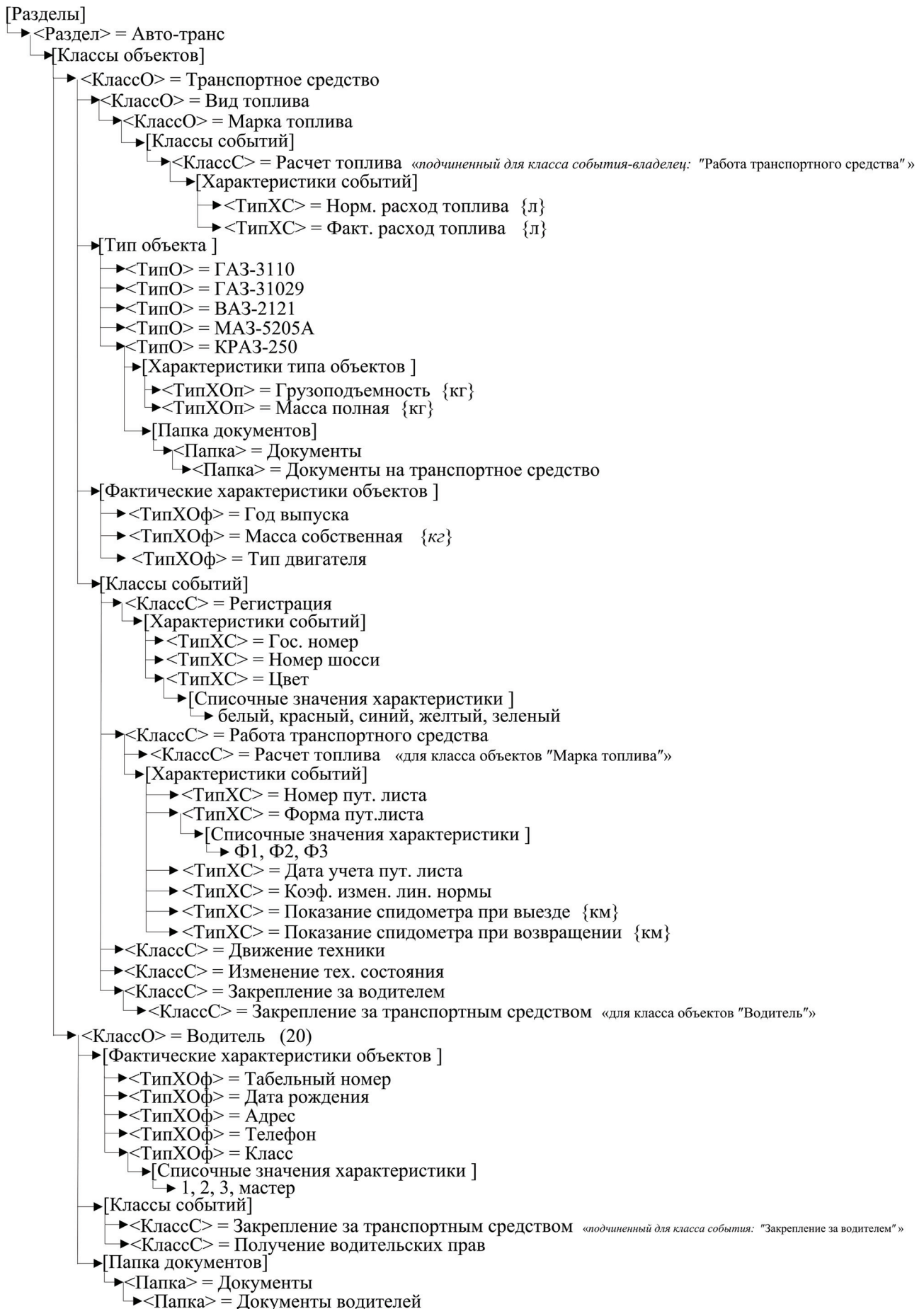
Рис. 5. Пример представления интенционала моделируемой ПрО
