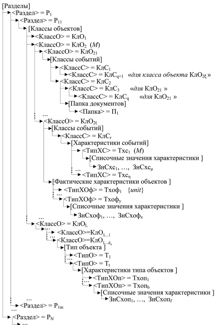
Рис. 4. Представление метаданных ПрО с помощью специальной формы записи ациклического ориентированного графа модели «объект-событие»
