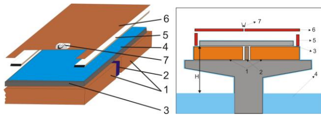
1 – измерительные электроды; 2 – заземленный электрод; 3 – диэлектрическая подложка; 4 – гелий; 5 – охранное кольцо; 6 – прозрачный для ИК излучения электрод; 7 – источник электронов Рис. 1
