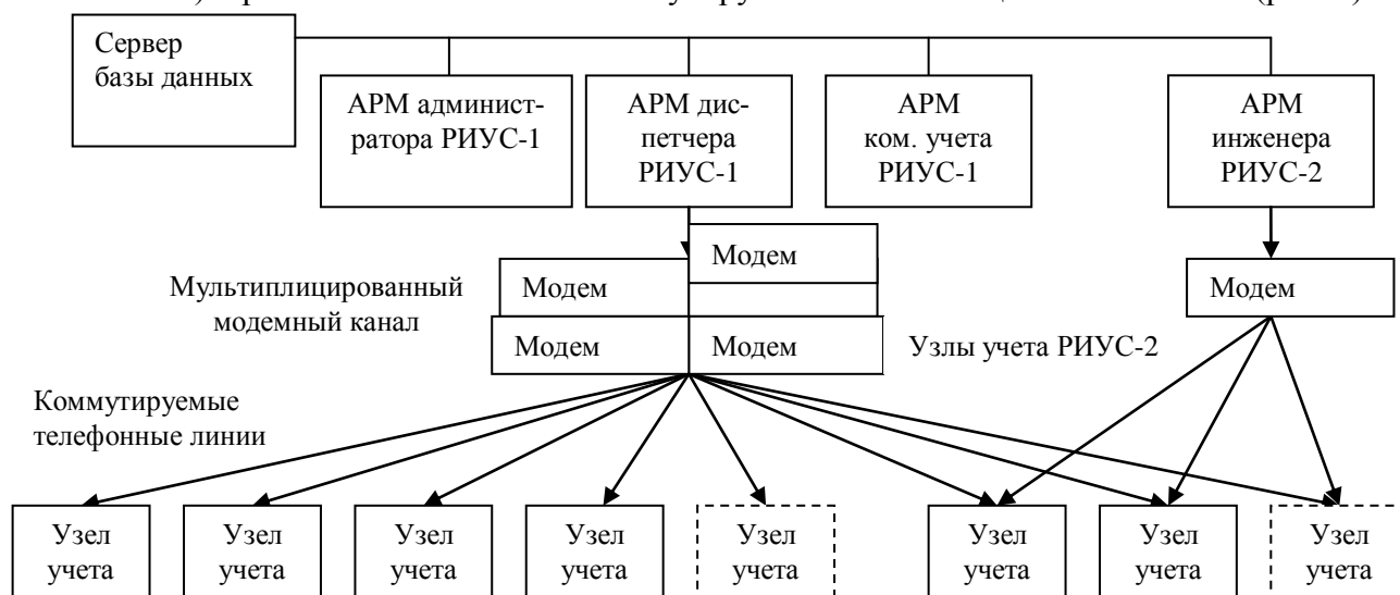
Рис. 1. Структура распределенных информационно-управляющих систем
