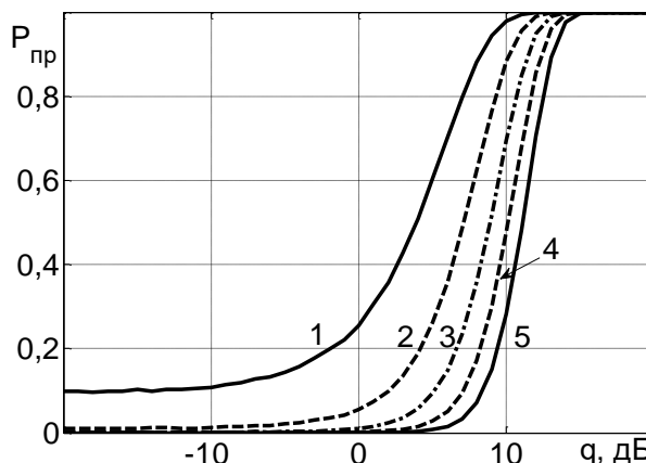
Рис. 3. Зависимость вероятности правильного приема от отношения сигнал/шум
