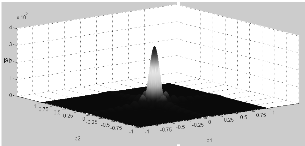
Рис. 7 Сигнальна функція S(q_1, q_2) при використанні простих зонduючих сигналів з прямокутними огинаючими
