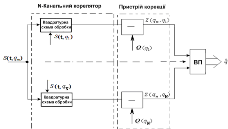
Рис. 1 Схема формування оцінок максимальної правдоподібності інформативного параметра в системах РАЗ
